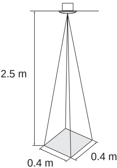
sensordetectiegebied voor enkele urinoir (125 sensor)
