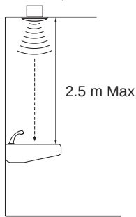
sensordetectiegebied voor enkele wasbakken (124 sensor)
