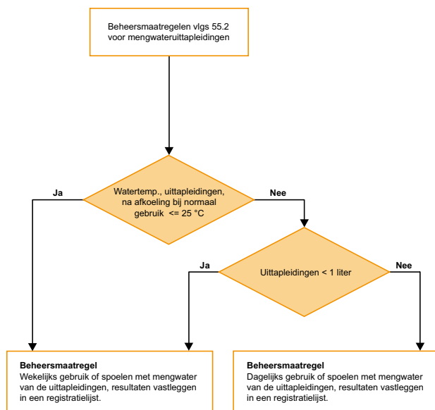
Stroomdiagram 2: beheersmaatregelen voor mengwater uittapleidingen vlg ISSO 55.2
