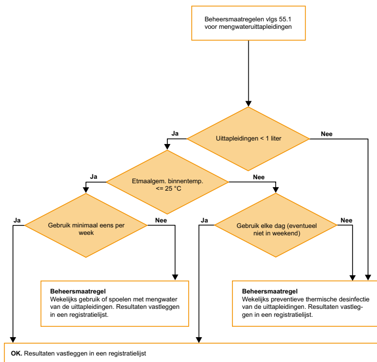
Stroomdiagram 1: beheersmaatregelen voor mengwater uittapleidingen vlg ISSO 55.1
