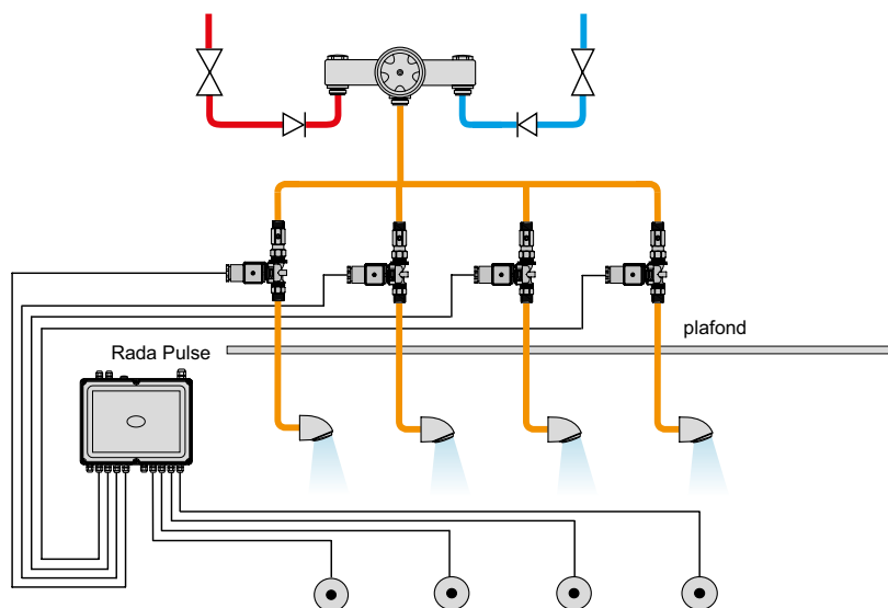
Rada Pulse douchebesturingssysteem met automatische cyclusspoeling aangesloten op een Rada centrale mengkraan
