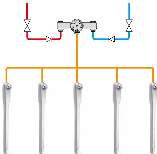
Meerdere Rada douchepanelen type Sport met automatische cyclusspoeling aangesloten op een Rada centrale mengkraan
