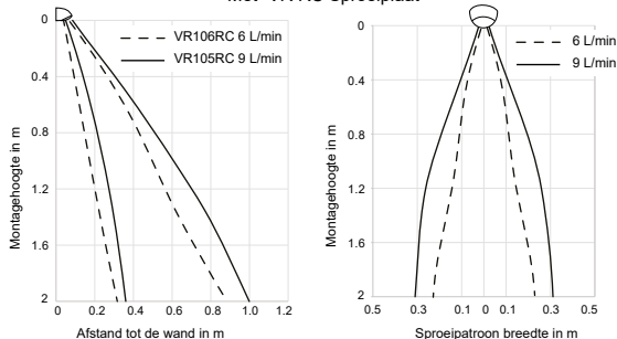
Sproeipatronen Met "VR RC Sproeiplateau"
