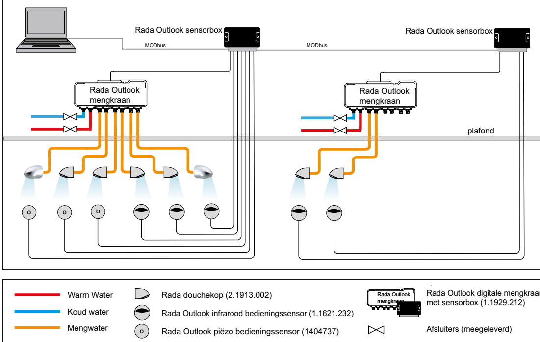
Meerdere Rada Outlook en Rada Outlook Duo digitale mengkranen met registratie van cyclusspoelingen
