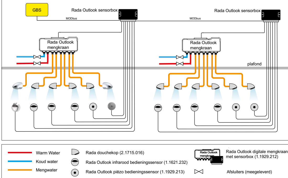
Meerdere Rada Outlook digitale mengkranen gekoppeld aan een GBS (MODbus)
