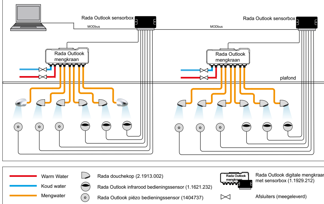
Meerdere Rada Outlook digitale mengkranen met registratie van cyclusspoelingen
