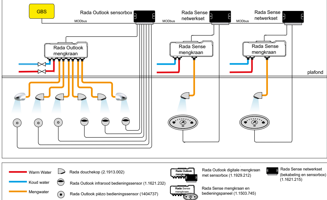
Meerdere Rada Outlook en Rada Sense digitale mengkranen gekoppeld aan een GBS (MODbus)
