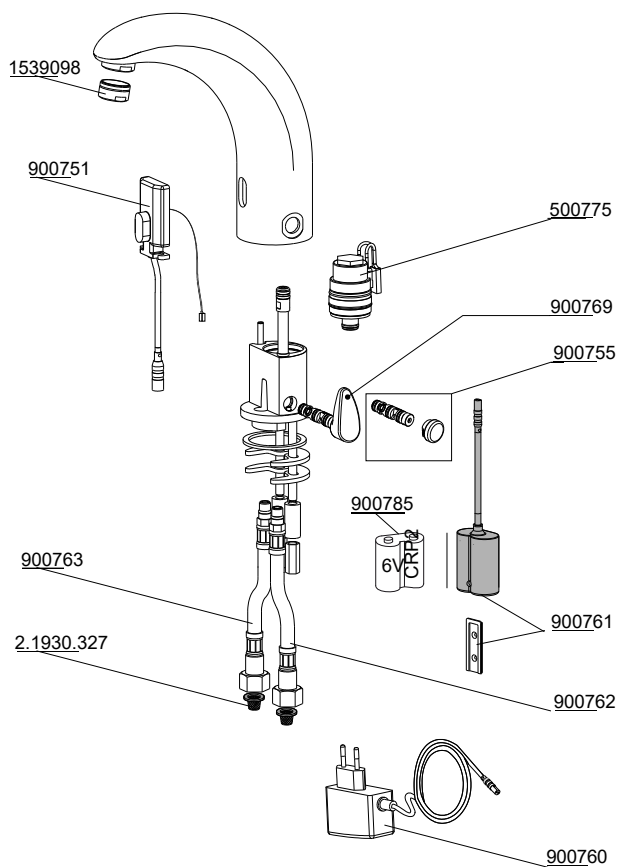
Rada Tec 100
